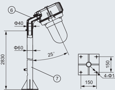
L: pole type 25°
