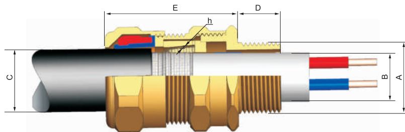
Cable wiring
