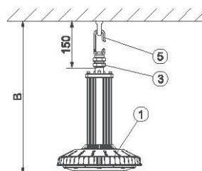
挂钩式(d) / Hook type (d)
