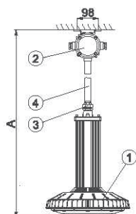
吊杆式 / Pendant pole type (g)
