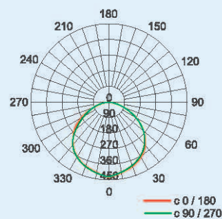
III 型 Type III
