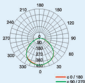
I 型 Type I
