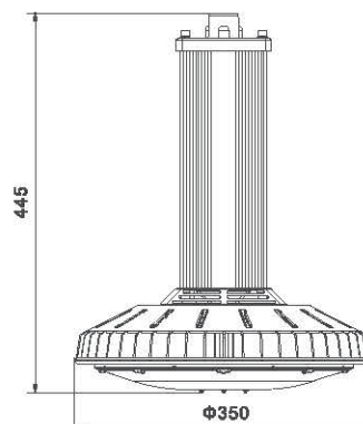
III 型 Type III
