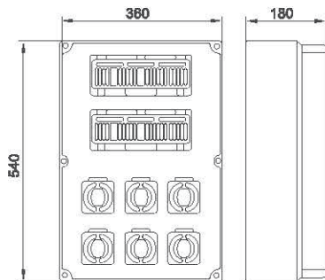
六回路/6 Circuits
