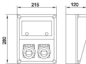
二回路/ 2 Circuits
