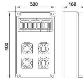
四回路/4 Circuits
